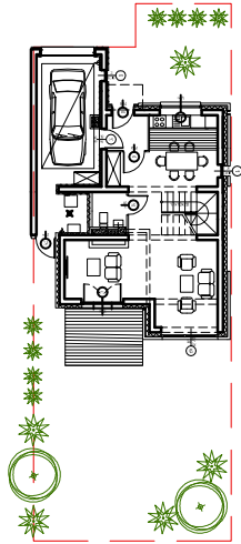
Rzut zagospodarowania działki
